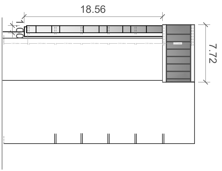
2 ELEVACION LATERAL DERECHA MURO CORTINA
